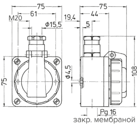
Чертеж 1 МВ 347 Размеры, мм.
