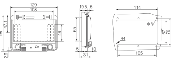
Шарнирное окно, 6 модулей
