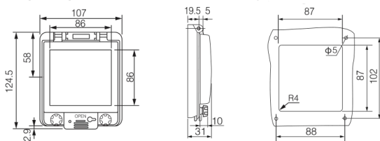
Шарнирное окно, 6 модулей
