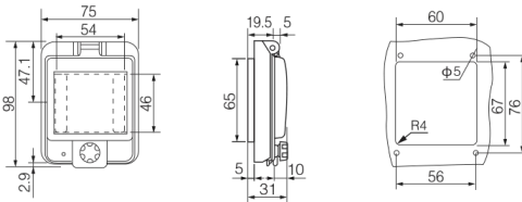
Шарнирное окно, 4 модуля
