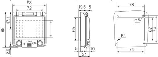
Шарнирное окно, 4 модуля
