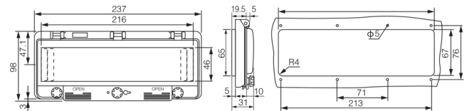
Шарнирное окно, 13 модулей
