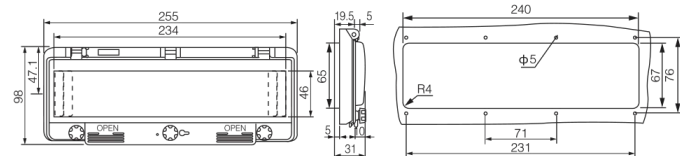
Шарнирное окно, 16 модулей
