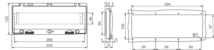
Шарнирное окно, 16 модулей
