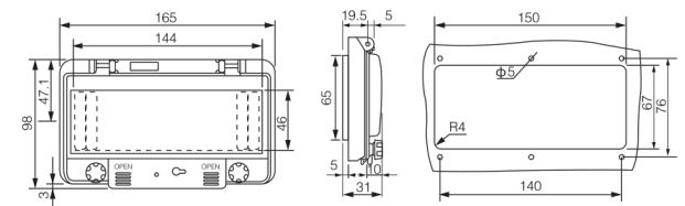
Шарнирное окно, 12 модулей
