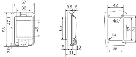
Шарнирное окно, 3 модуля
