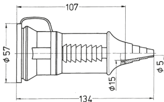
Чертеж 3 МВ 39 Размеры, мм.
